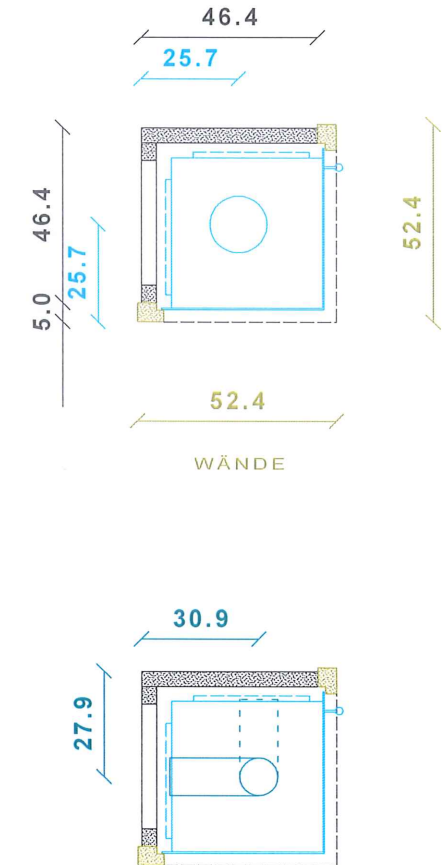
Verbrennungsluftzufuhr 100mm DM
